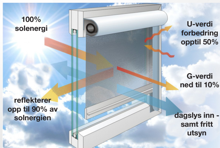
Multifilm solskjermingssystem med transparent og høyreflektiv film.
